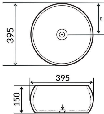
Umywalka nablatowa ALICE
