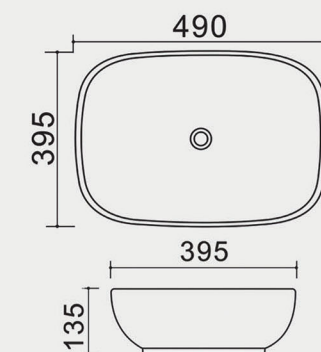
Umywalka nablatowa NILA
