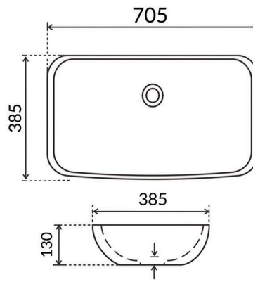
Umywalka nablatowa ISMENA 70
