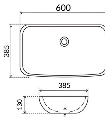
Umywalka nablatowa ISMENA 60
