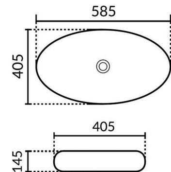
Umywalka nablatowa LEA
