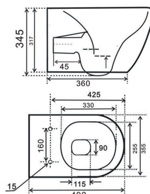
Miska wisząca FERRIS BEZ KOŁNIERZA
