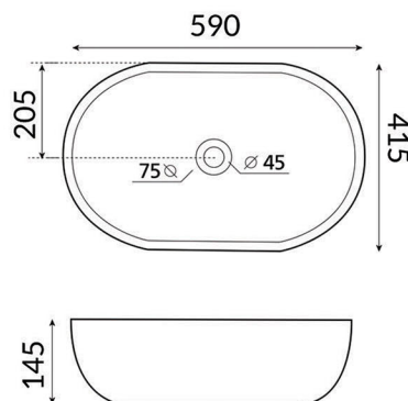
Umywalka nablatowa GRETA
