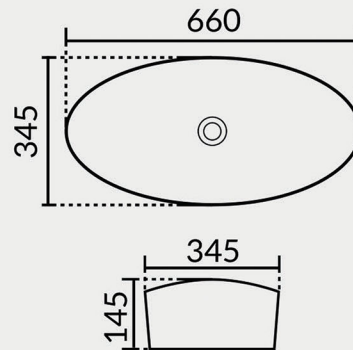
Umywalka nablatowa LATIKA
